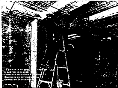
Instalación de tubería EMT para luminarias nivel 3.
